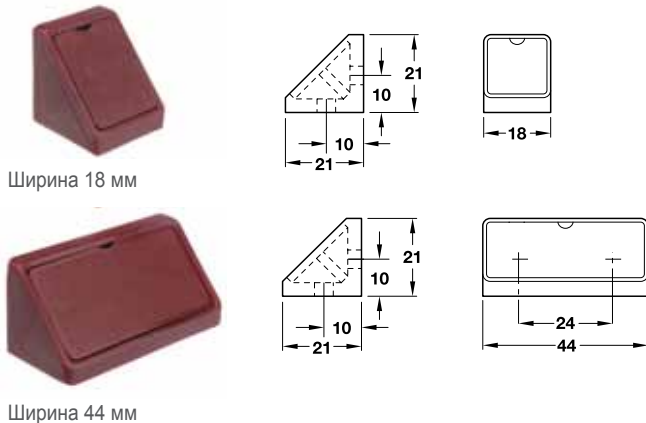
Ширина 44 мм
